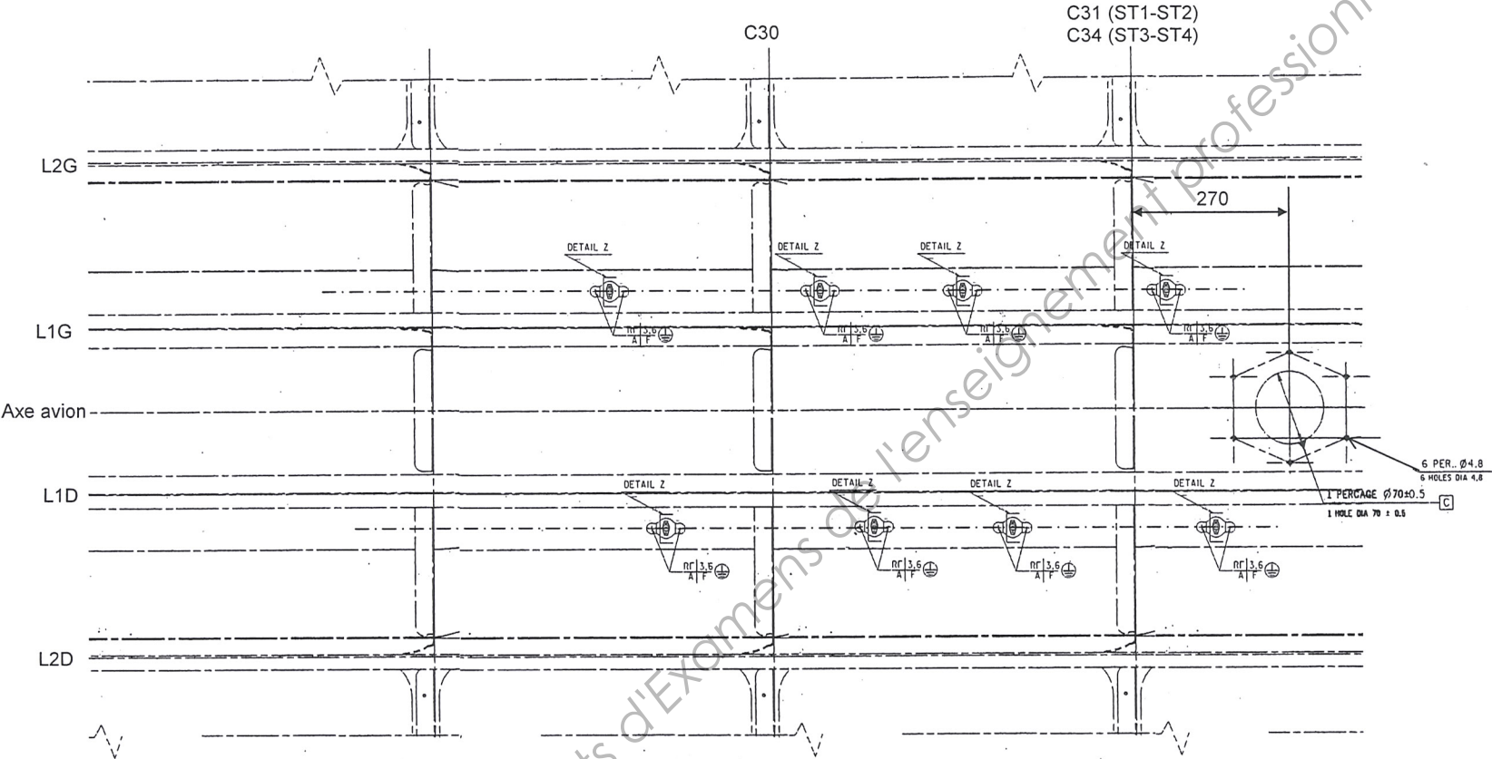
Détail Z
