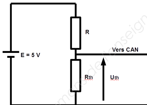
Figure 2 : schéma du montage potentiométrique
